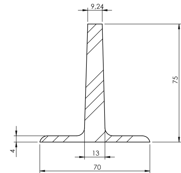
SEZIONE A-A
